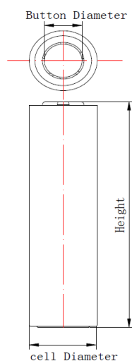
Cell 1 (IMR18650-1500mAh)
